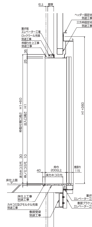
出入口断面图
