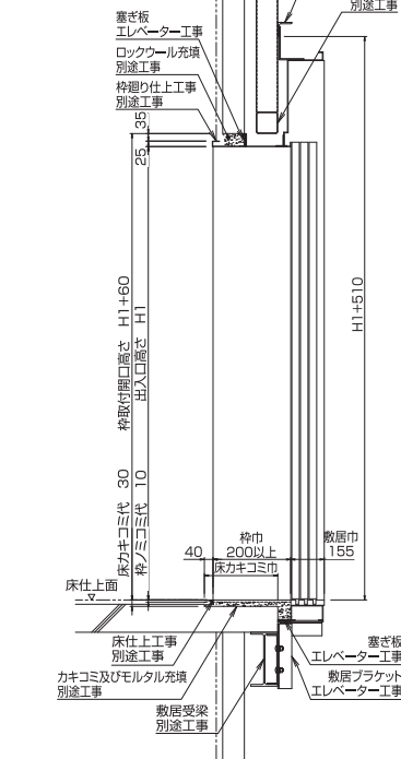
出入口断面图
