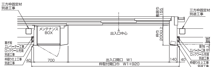
出入口平面図(最下階)
