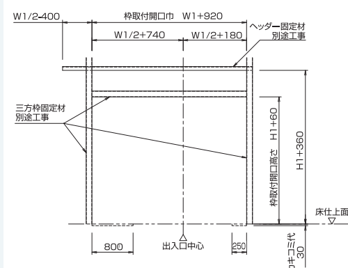
出入口穴あけ図(最下階)
