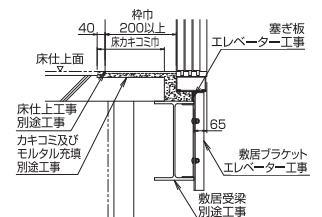
積載2,000kg超えの 敷居下部断面図
