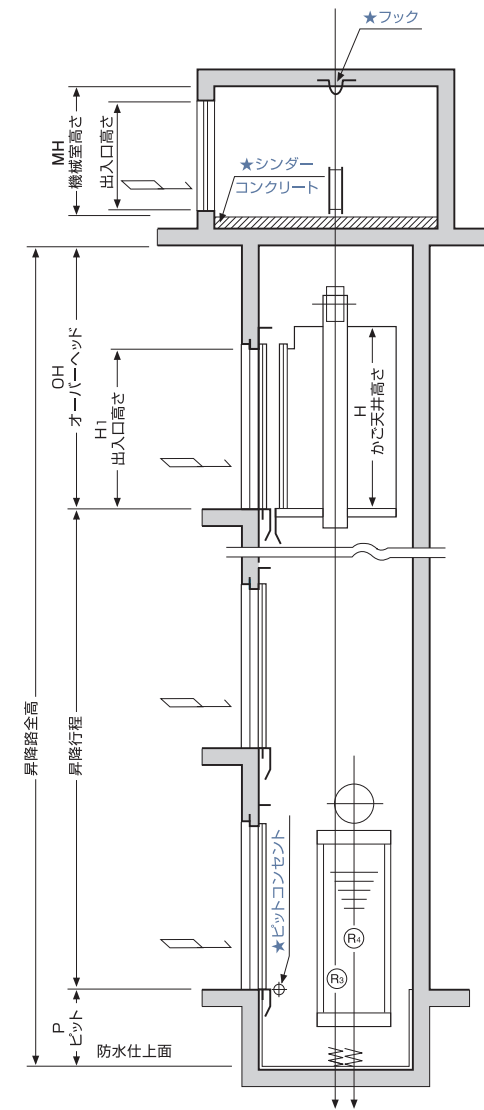
昇降路縦断面図
