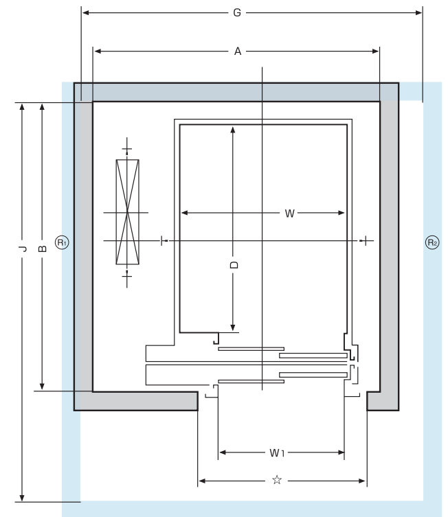
昇降路／機械室平面図
