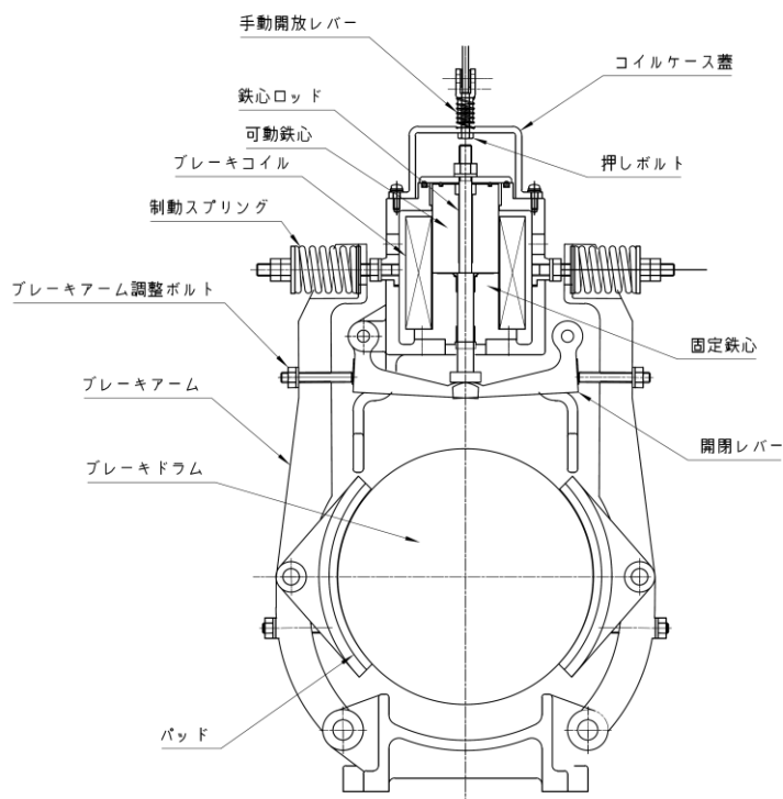
図 2: ダブルスプリングブレーキ構造図手動開放レバー有り
