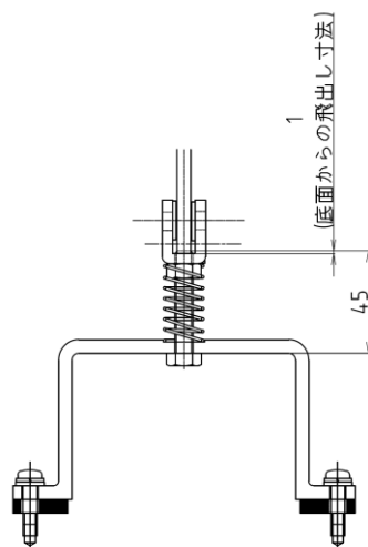
押しボルト M8X45の取付寸法拡大図
