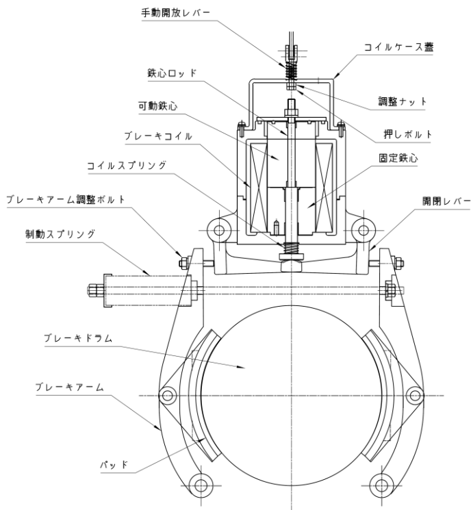
図1: シングルスプリングブレーキ構造図手動開放レバー有り
