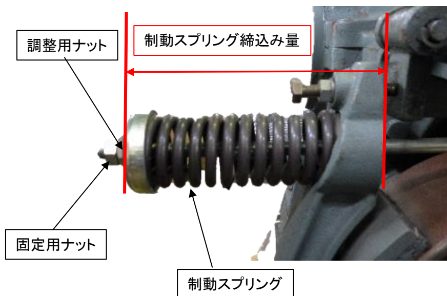
図6 ： 制動スプリングセット位置
