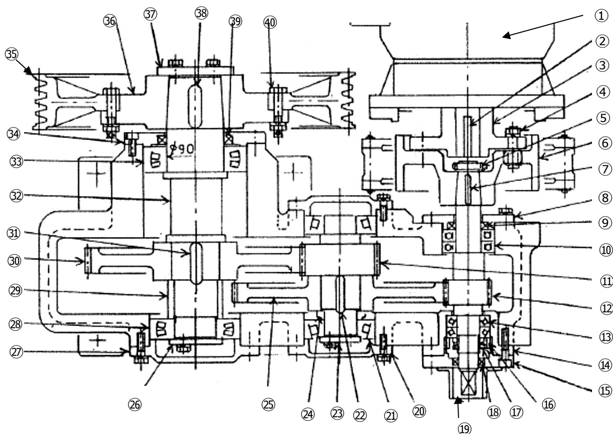
図10-1 構造図 ヘリカルギヤ式トラクションマシン (スタンド無しの例)
