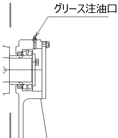
図 2 スタンド部グリース注油口
