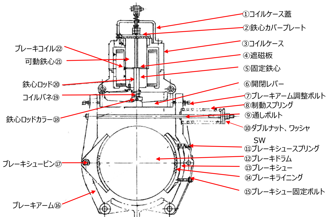
図3：ダブルスプリングブレーキ構造図
