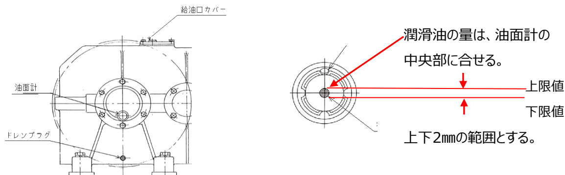
図 1 : 給廃油口
