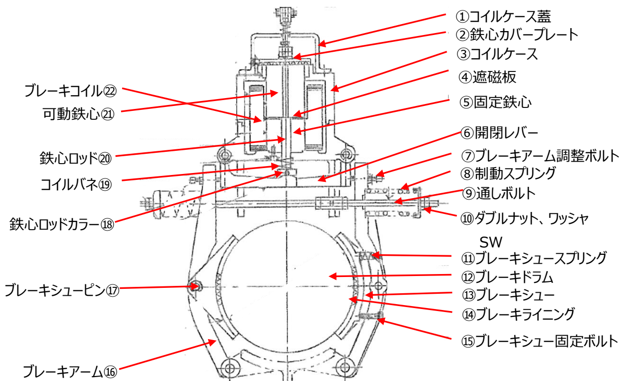
図3：ダブルスプリングブレーキ構造図
