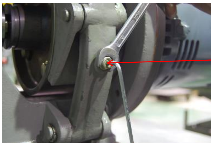
写真 6 ブレーキシュー固定ボルト
