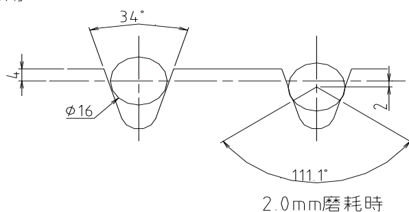
図 9 : V溝寸法及び摩耗時、アンダーカット角
