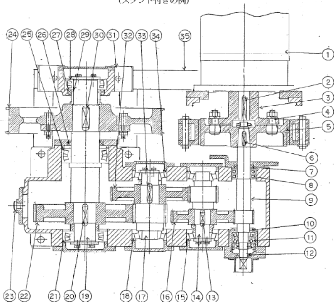
図10-3 構造図 ヘリカルギヤ式トラクションマシン (スタンド付きの例)
