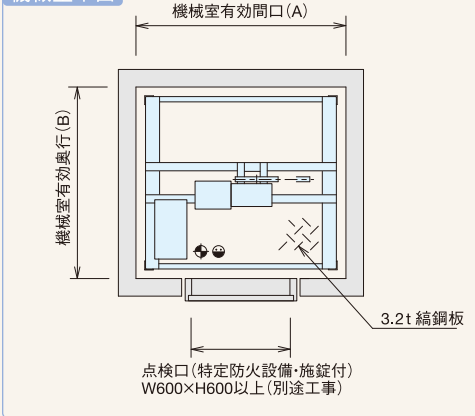
機械室平面
