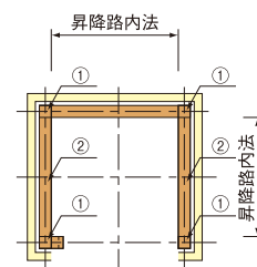
昇降路平面
