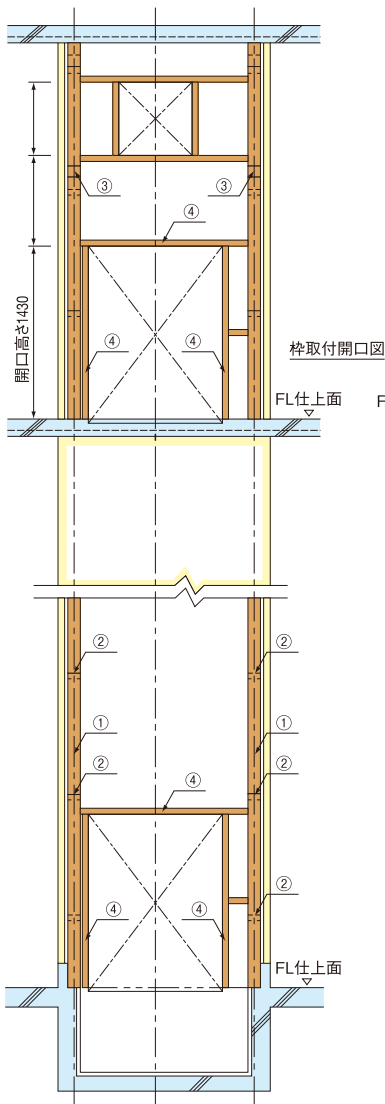
昇降路断面（正面）
