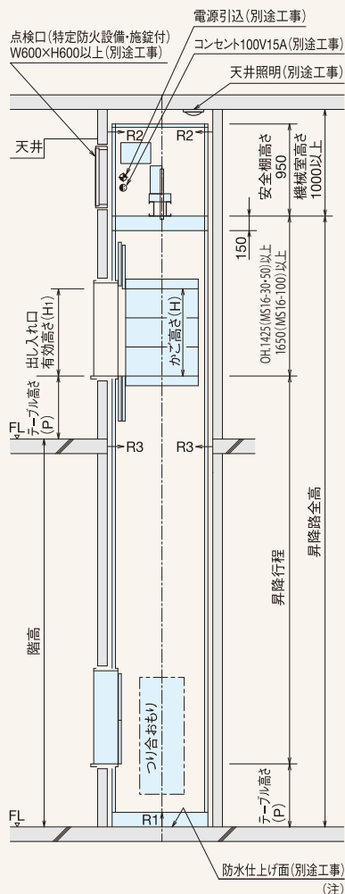
昇降路断面
