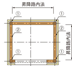
昇降路平面
