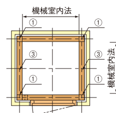
機械室平面
