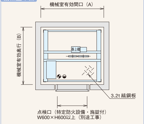
機械室平面
