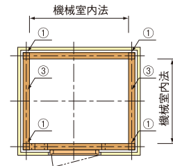
機械室平面
