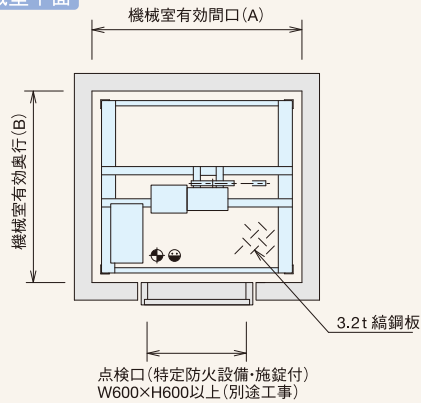
機械室平面
