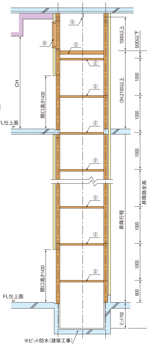
昇降路断面（側面）
