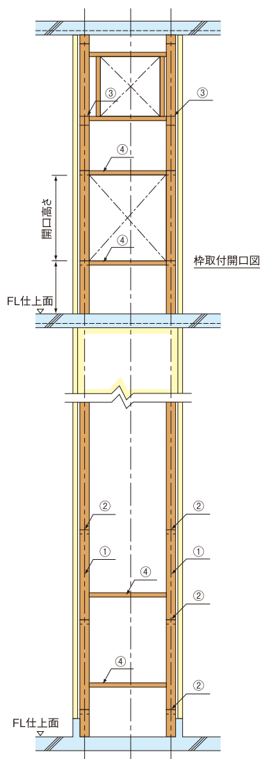
昇降路断面（正面）
