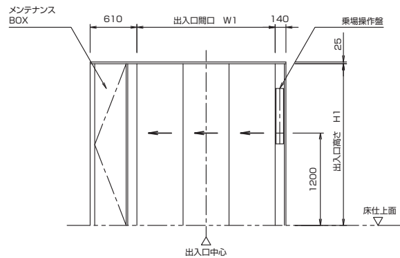
出入口正面図 (最下階)
