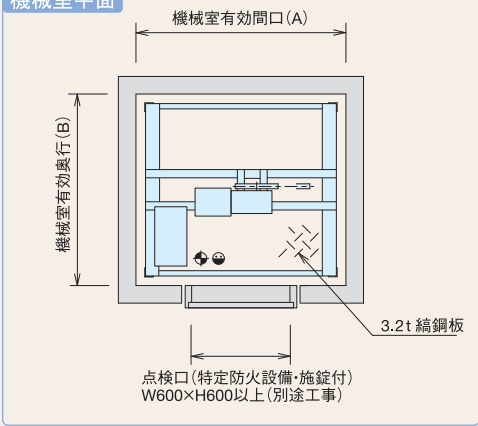
機械室平面
