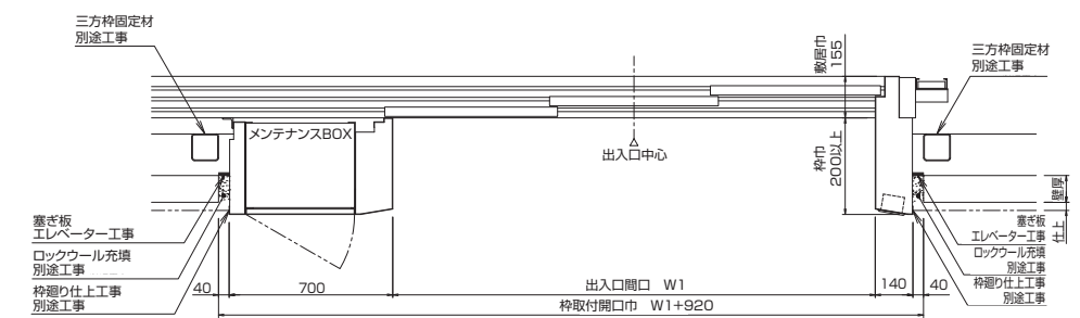
出入口平面図(最下階)
